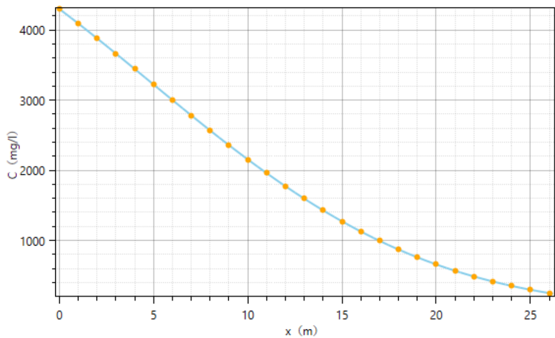
图 6.5-5 持续泄露 5a 不同距离地下水 COD Mn 浓度
