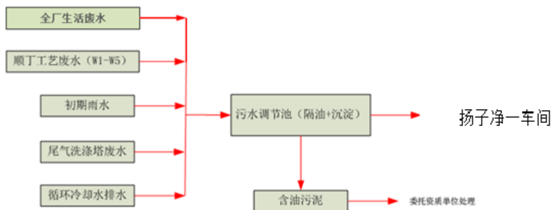
图 3.2.4-2 顺丁污水预处理站工艺流程图
