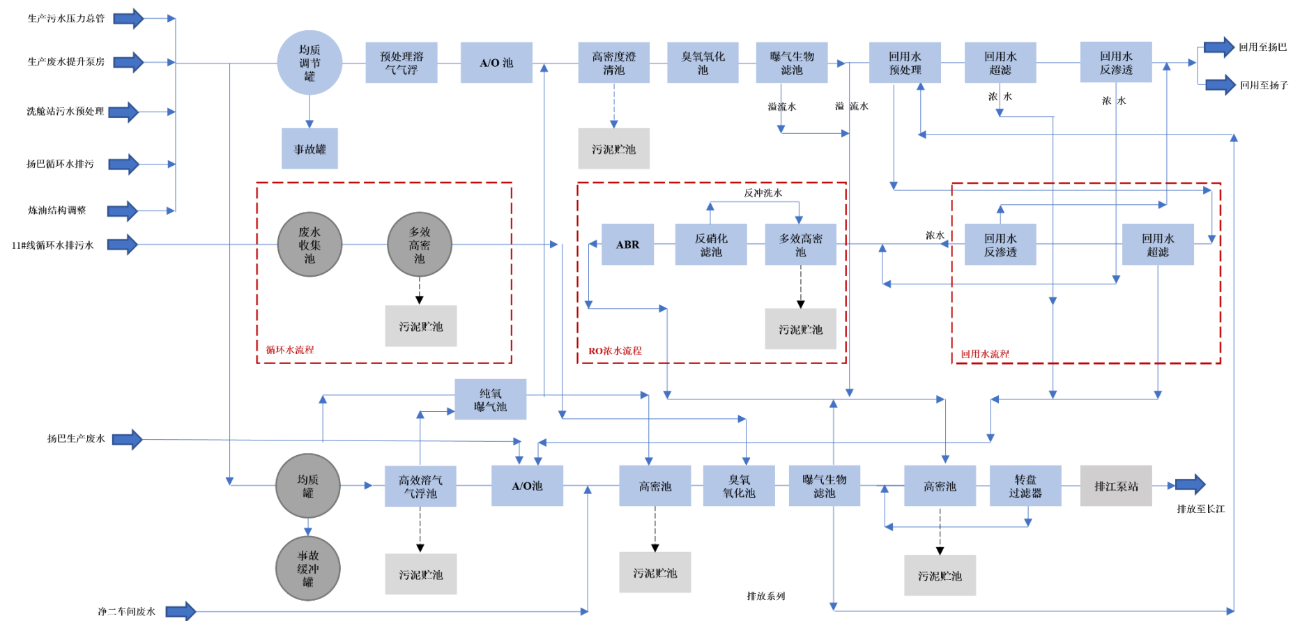
图 3.2.4-3 净一车间工艺流程图
