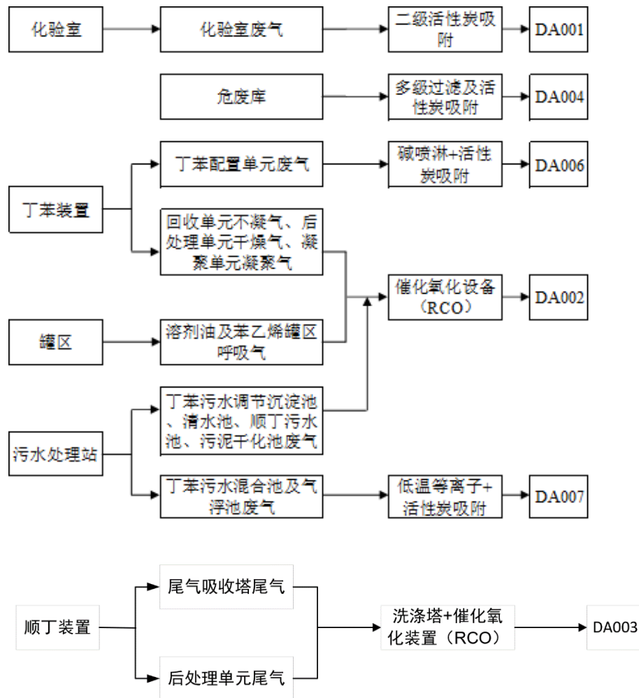
图 3.2.4-5 橡胶厂废气治理措施
