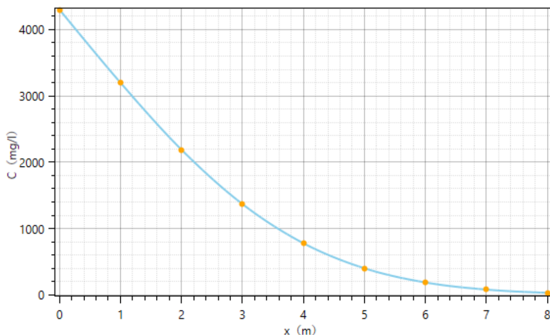
图 6.5-2 持续泄露 100d 不同距离地下水 COD Mn 浓度
