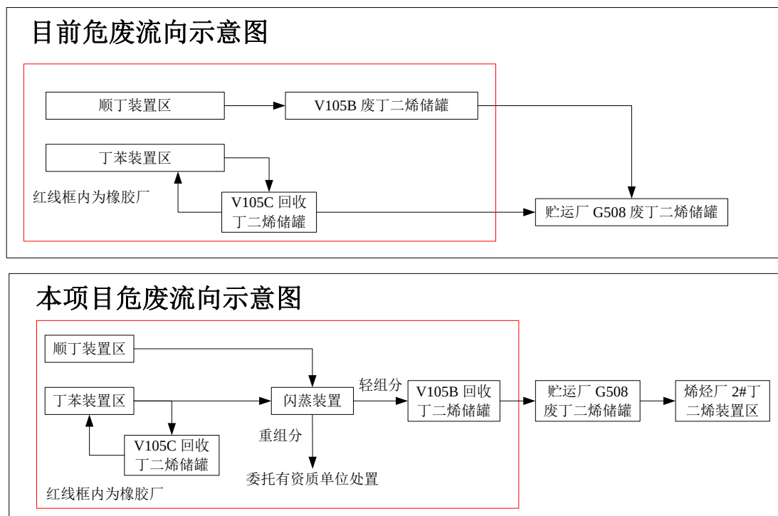
图 4.1-1 本项目危废综合利用流向路线图
