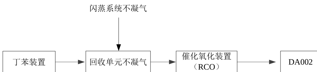
图 7.1-1 有组织废气处理整体流程示意图
