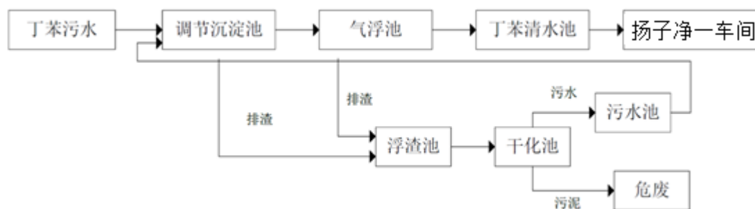
图 3.2.4-1 丁苯污水预处理站工艺流程图
