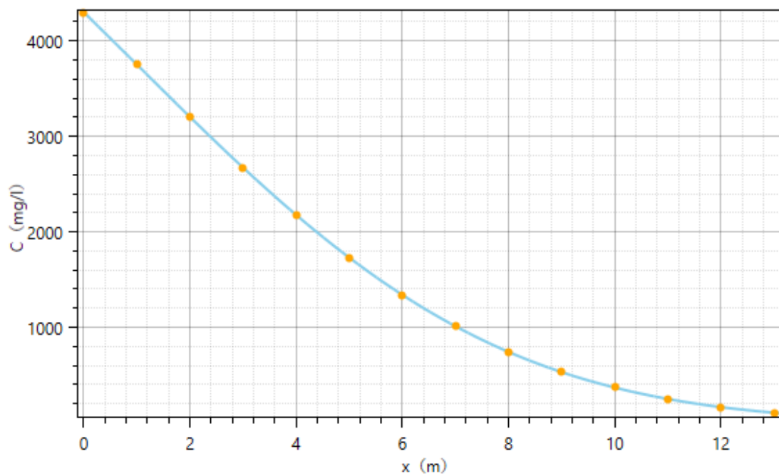
图 6.5-3 持续泄露 1a 不同距离地下水 \text{COD}_{\text{Mn}} 浓度
