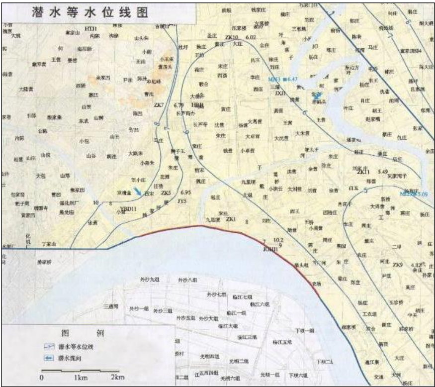
图 5.2-5 评价区地下水等水位线图
