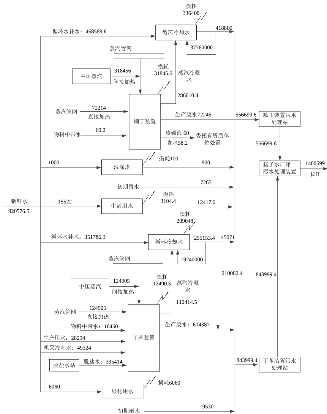
图3.2.4-4 现有项目水平衡图
