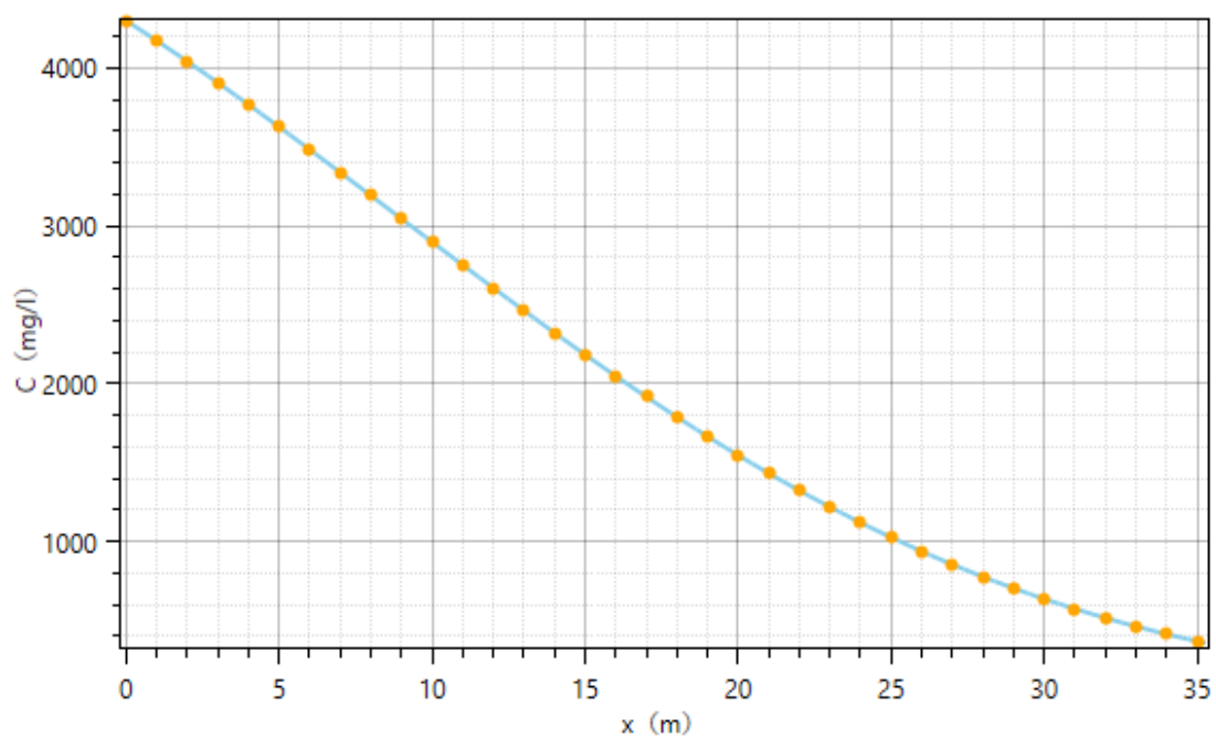
图 6.5-6 持续泄露 10=0a 不同距离地下水 COD Mn 浓度
