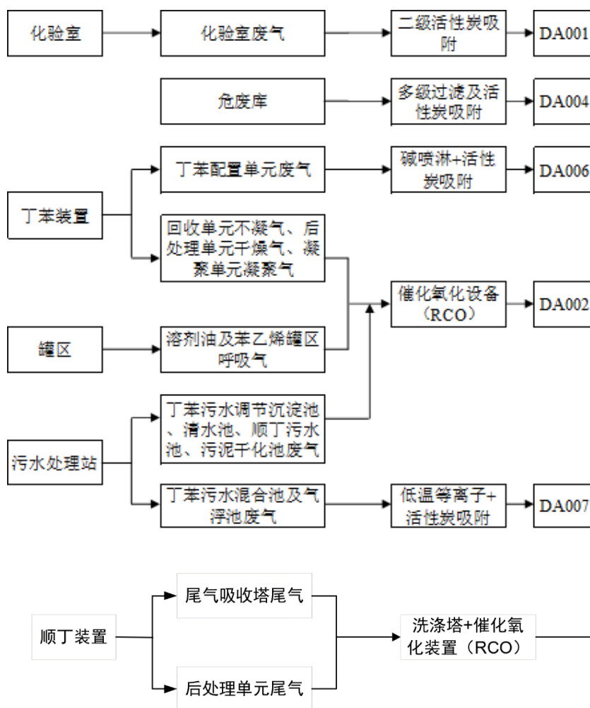
图 7.1-2 技改后全厂有组织废气处理整体流程示意图
