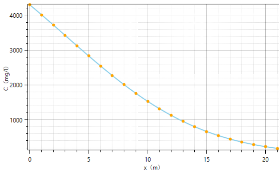
图 6.5-4 持续泄露 3a 不同距离地下水 \text{COD}_{\text{Mn}} 浓度
