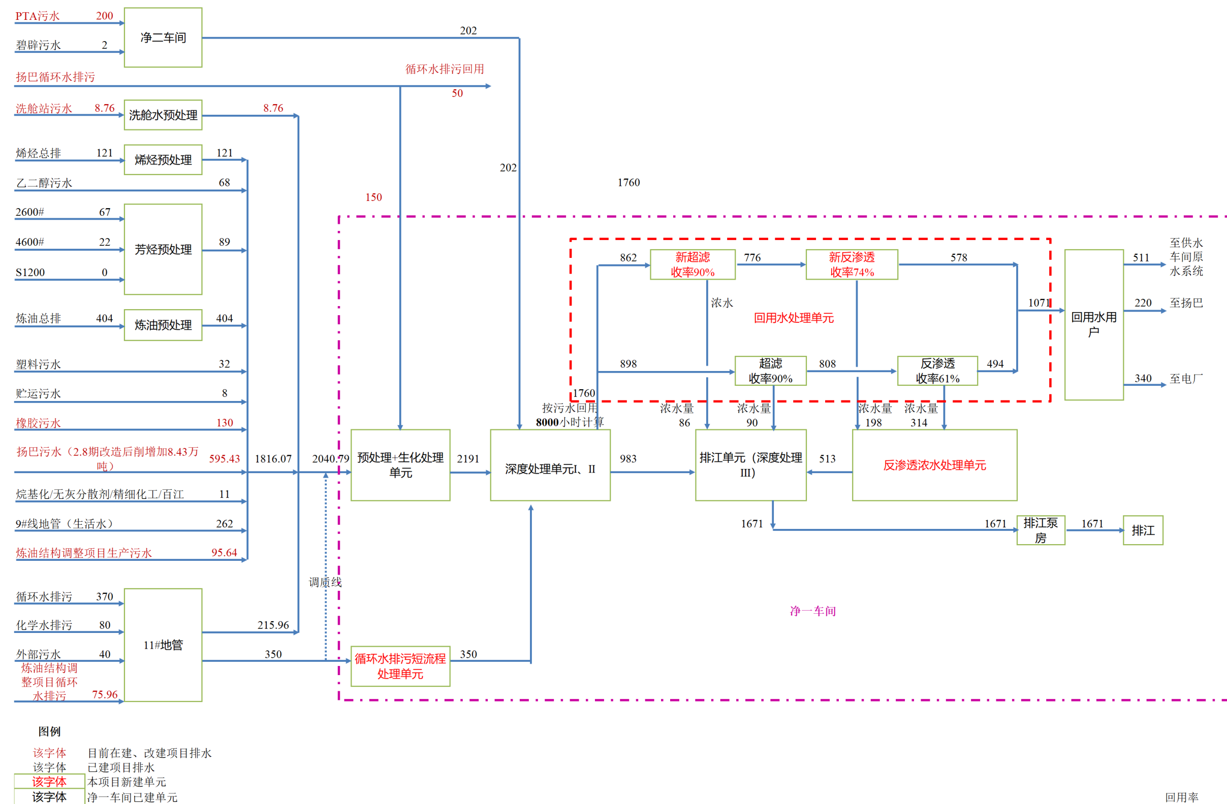
图 3.1-2 扬子石化循环水排污水处理及节水减排项目建成扬子石化水平衡图
