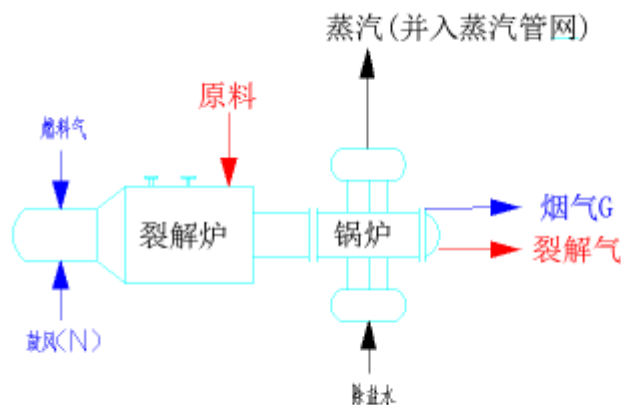
图 5-1 项目工艺流程图
