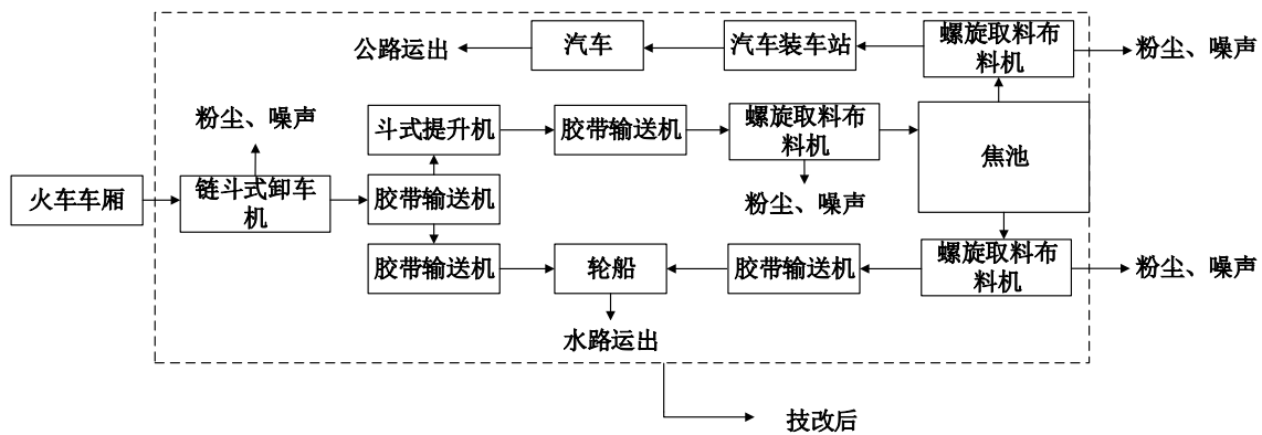
图4 项目改造后营运期工艺流程图
