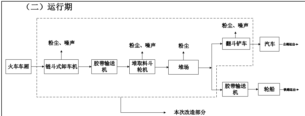
图3 项目改造前营运期工艺流程图
