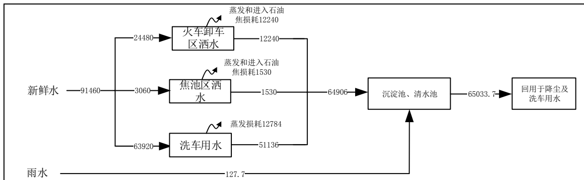
图 5 技改后用排水平衡图 单位: t/a
