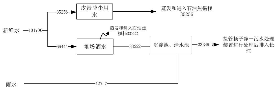
图1 技改前用排水平衡图 单位: t/a
